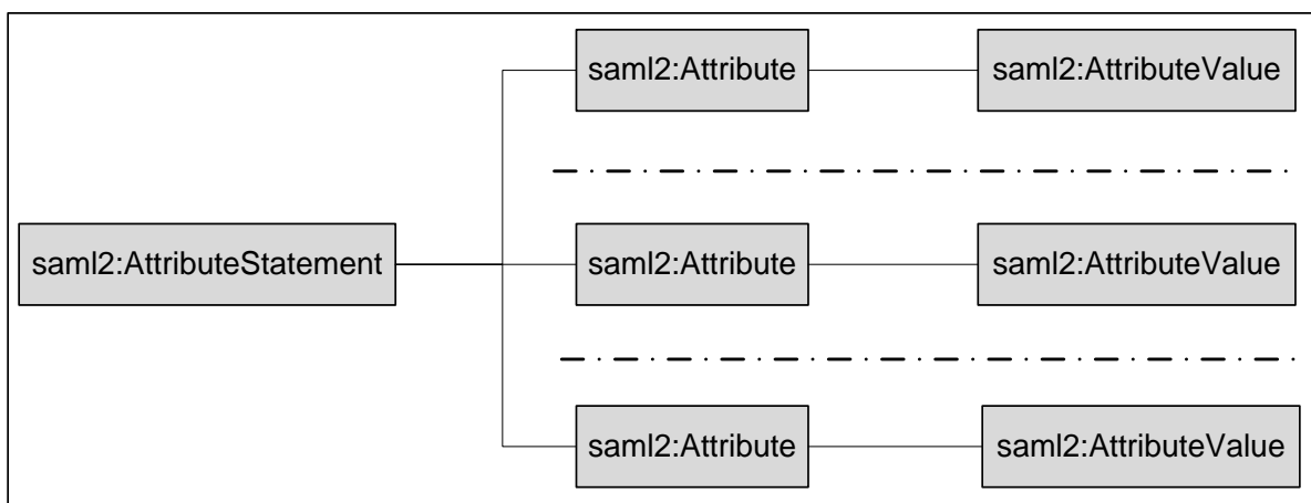
Рисунок 10 – Структура saml2:AttributeStatement
